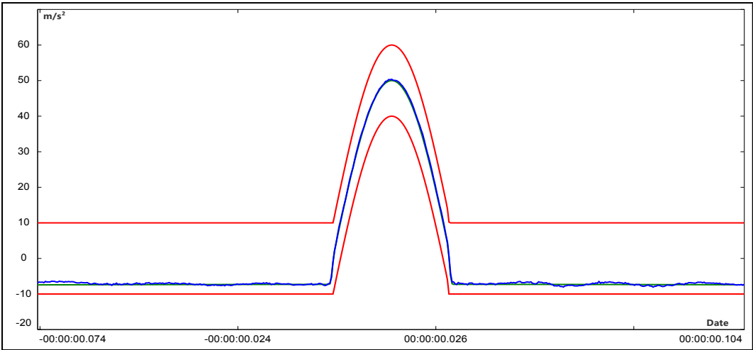
图 4 冲击试验
